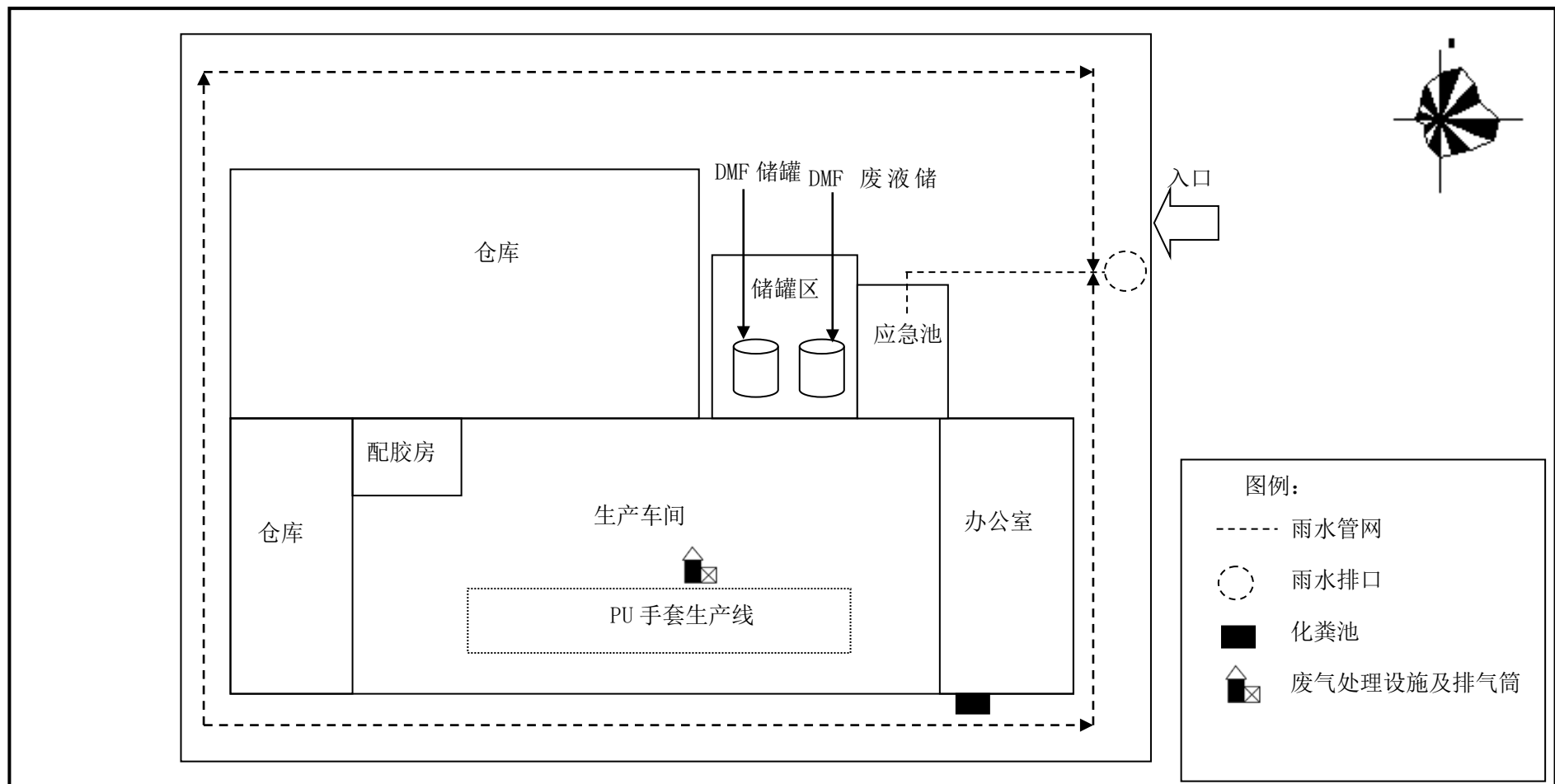
图 2-2 平面布置图
